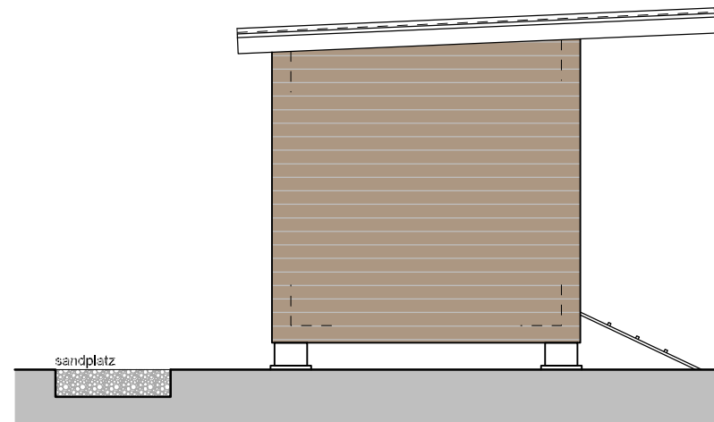
ansicht west
