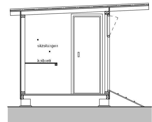
schnitt
