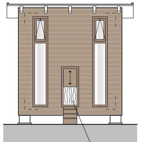
ansicht süd
