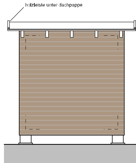
ansicht nord
